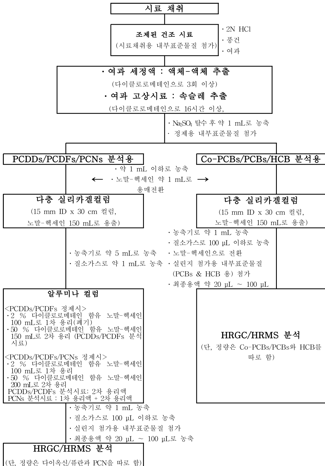
그림 1. 토양/퇴적물 시료 중 비의도적 잔류성유기오염물질 전처리 흐름도
